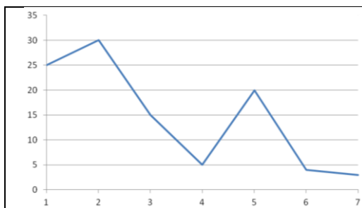
Liniendiagramm
