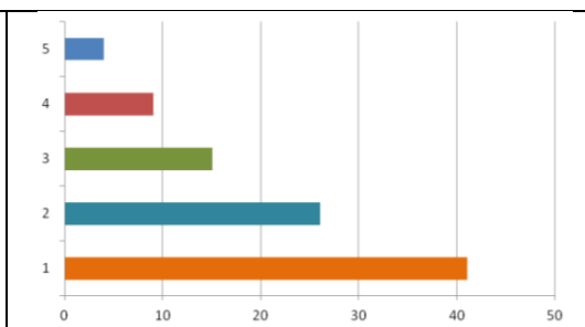
Balkendiagramm
