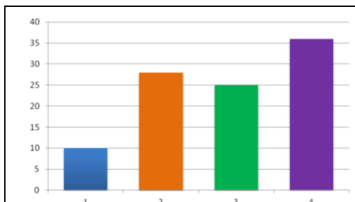
Säulendiagramm
