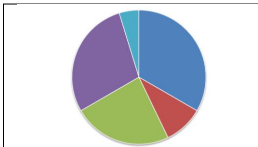
Kreisdiagramm
