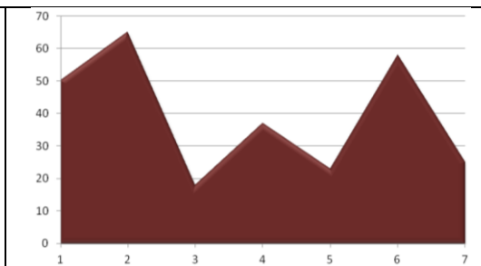
Flächendiagramm
