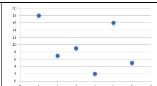
Punktdiagramm
